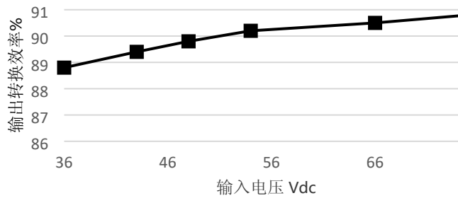
输入电压降额曲线
