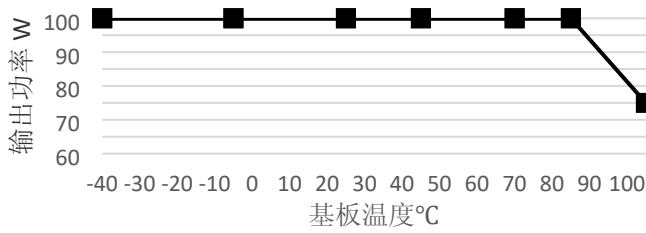
48V 输入降额曲线图
