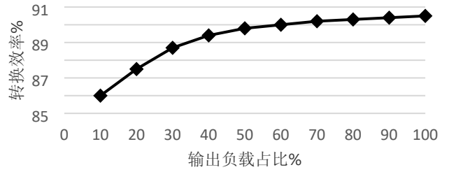
负载效率曲线
